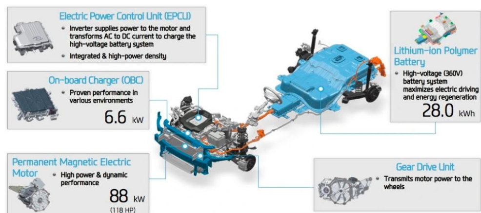
圖 14：傳統電動車分離式部件
