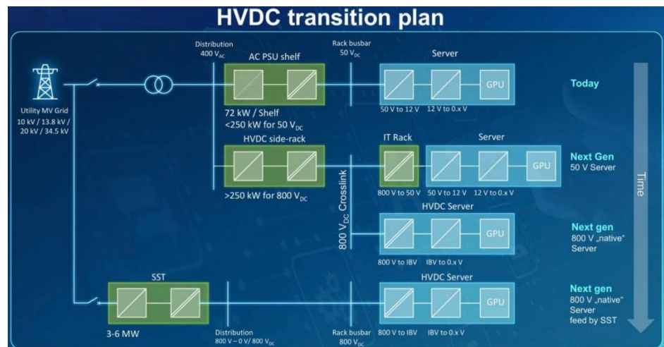
圖 7：電源架構趨勢明確，產值持續提升。台達電擁電網-電力傳輸-伺服器至板上電力解決產品
